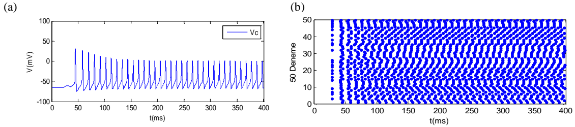
Şekil 5. MTF11’de C hüresine (uyarım-E) seçilerek, A hüresine Şekil 2.a’deki akım uygulandığında (a) C hüresinde oluşan aksiyon potansiyelleri (b) 50 deneyin her biri için C hüresinde aksiyon potansiyeli tepe değerlerinin zamanları.
