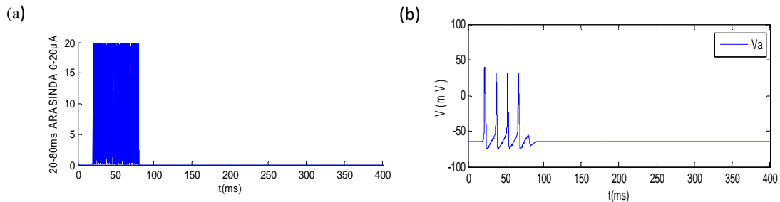
Şekil 2. (a) 0 – 20 \mu A düzgün dağılımlı rastlantısal akım, Şekil 1-a'daki hücre modeline uygulandığında (b) hücre modelinin ürettiği aksiyon potansiyelleri dizisi.
