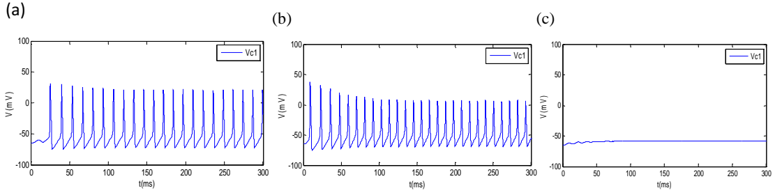
Şekil 4. MTF1’de 10\mu A ’lık DC akım (a) A hüresine (b) A ve B hücrelerine (uyarım, AB-EE) (c) A ve B hücrelerine (uyarım, AB-EI) uygulandığında, C hüresinin cevabı.
